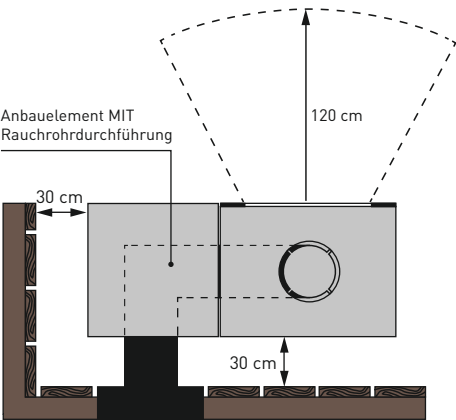
Draufsicht Brennkammer
