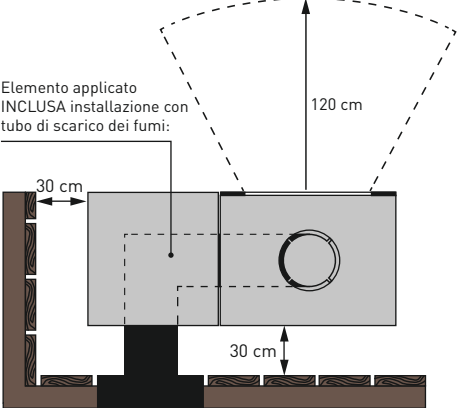
Vista dall'alto
