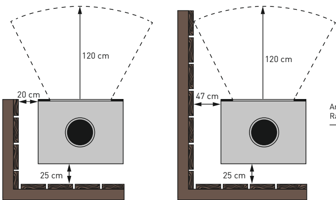
Draufsicht Brennkammer
