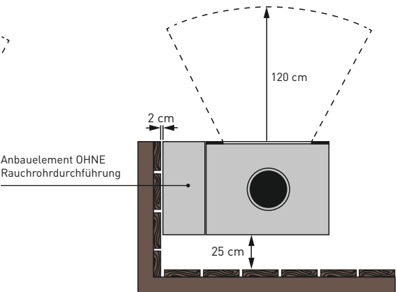
Draufsicht Brennkammer
