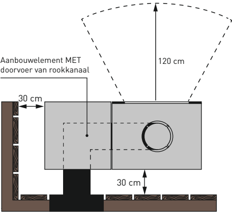
Bovenaanzicht
