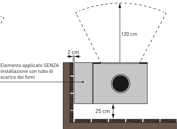
Vista dall'alto
