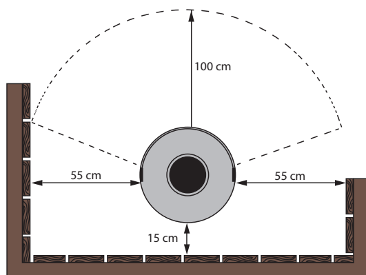
Draufsicht Brennkammer
