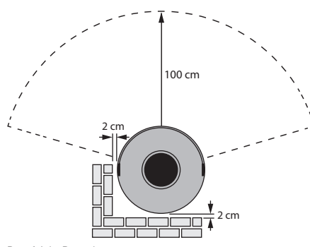
Draufsicht Brennkammer
