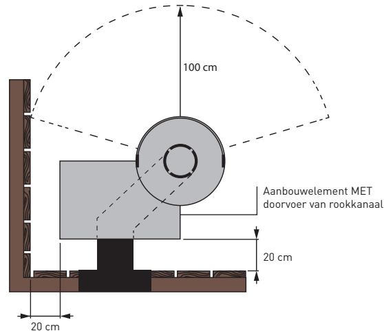
Bovenaanzicht
