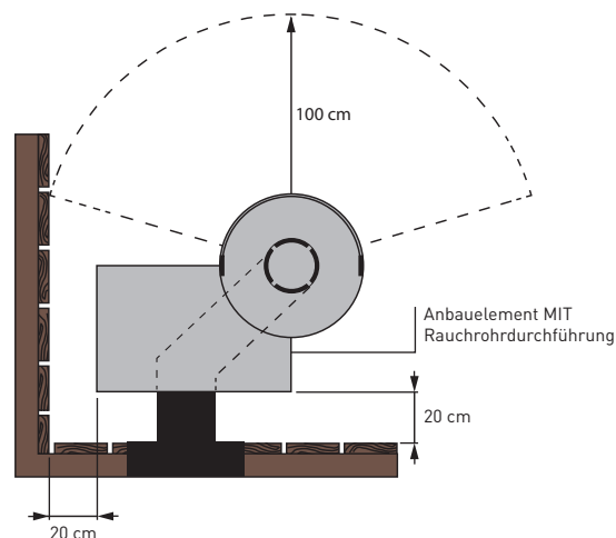
Draufsicht Brennkammer
