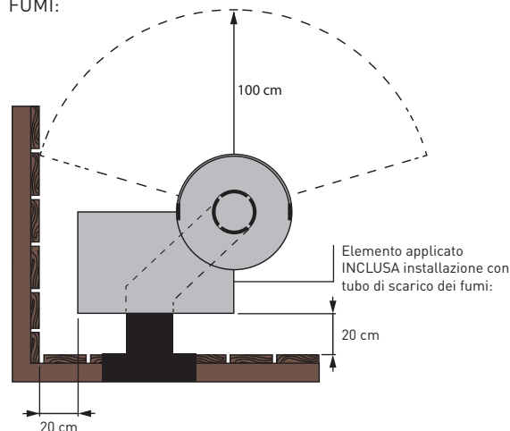
Vista dall'alto
