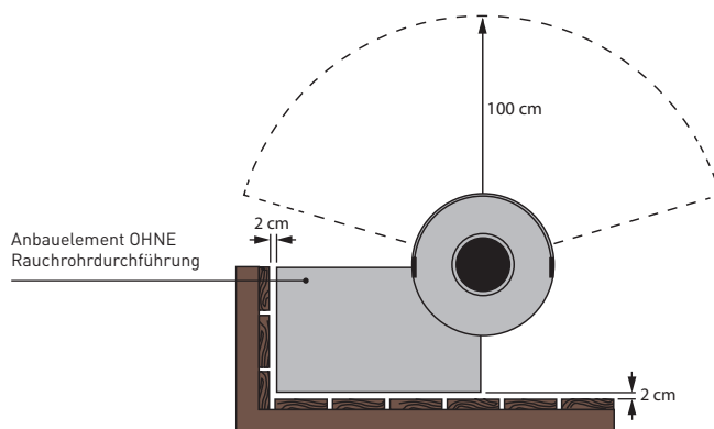
Draufsicht Brennkammer
