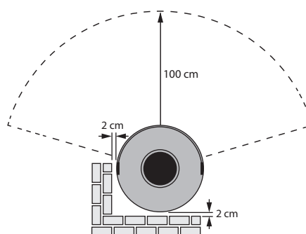
Vista dall'alto
