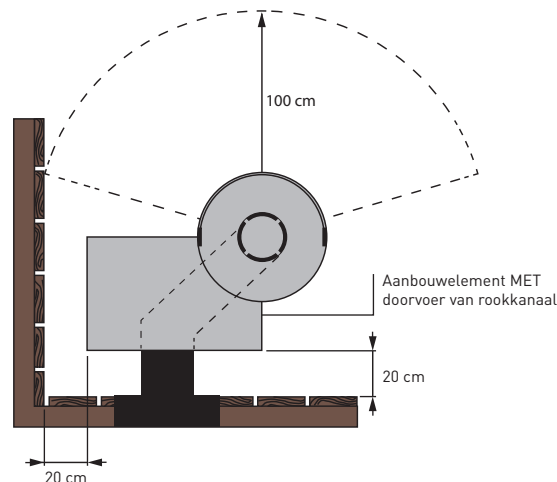
Bovenaanzicht
