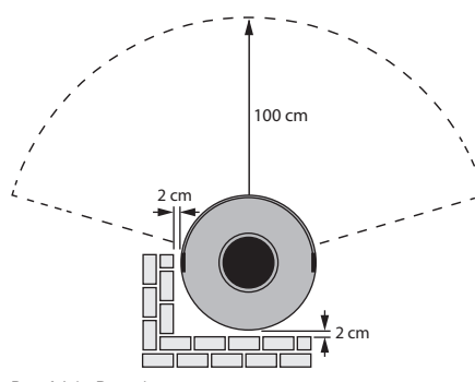
Draufsicht Brennkammer
