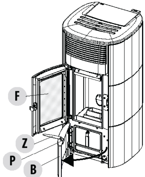
ÖFFNEN DER UNTEREN TÜR
